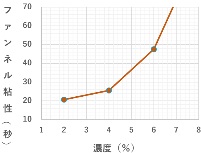
ファンネル粘性と濃度
